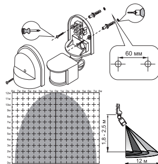
Schemat obszarów krycia czujnika (180°): Strefa wykrywania i aktywacji
